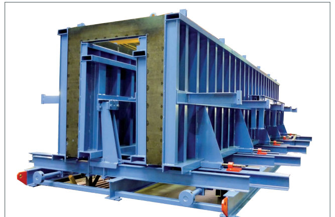
Канал для прокладки кабеля U-образной формы
