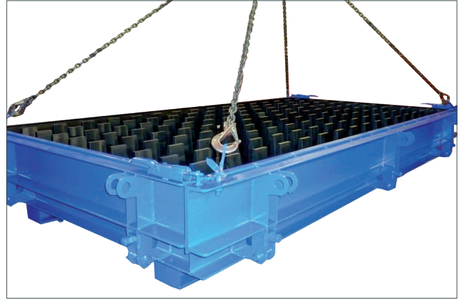
Płyta kratkowa
