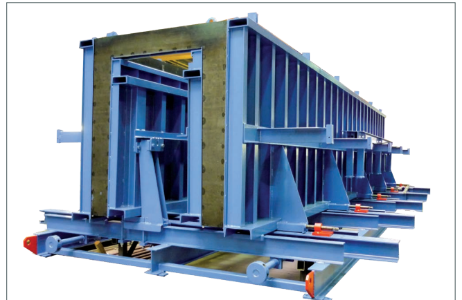
U型管道构件
