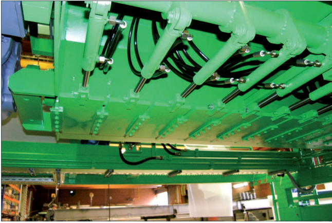
平推仓口滚轮式布料机
