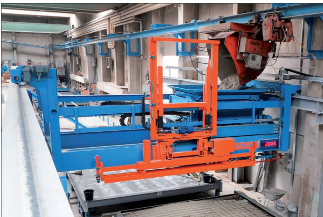
Abziehvorrichtung am Betonverteiler
